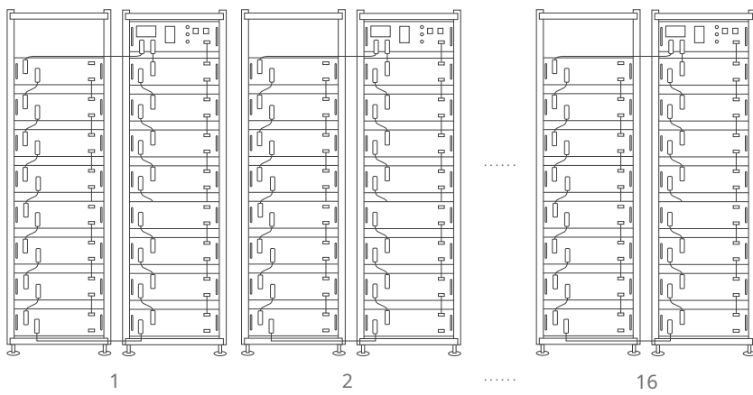
Максимална поддръжка за 16 клъстера батерии, свързани паралелно
